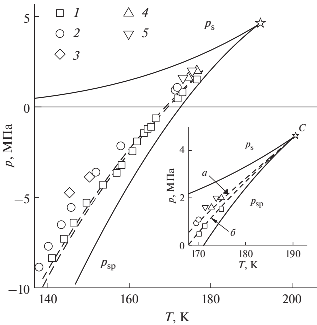
Рис. 2. Предельные растяжения ( J=10^{21} \text{ м}^{-3} \text{ с}^{-1} ) метана (1) и раствора метан–гелий (2) – c = 0.1 и (3) – 0.2 моль %). Точки – эксперимент, штриховые линии – КТЗ (нижняя – метан, верхняя – раствор, метан–гелий, c = 0.1 моль %). p_s – линия насыщения, p_{sp} – спинодаль, C – критическая точка. На вставке рисунка: предельные растяжения ( J = 10^7 \text{ м}^{-3} \text{ с}^{-1} ) метана (4) и раствора метан–гелий (5– 0.1 моль %) [10]. Штриховые линии – КТЗ, чистый метан ( a - J = 10^7 \text{ м}^{-3} \text{ с}^{-1} , b - J = 10^{21} \text{ м}^{-3} \text{ с}^{-1} ).
