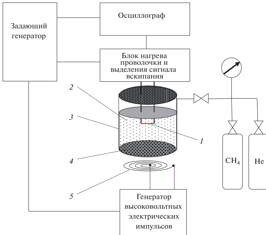
Рис. 1. Схема экспериментальной установки: 1 – платиновая проволочка d = 20 мкм, l = 1 см, 2 – жидкость V = 50 см 3 , 3 – камера, 4 – дюралевая мембрана, 5 – плоская катушка.
