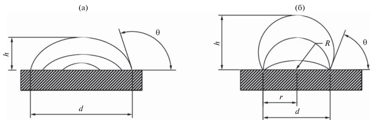
Рис. 4. Схематичное изображение роста незакрепленного (а) и закрепленного (б) сидящего пузырька.
