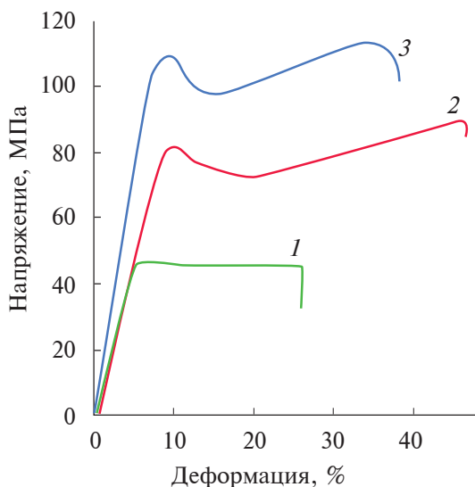
Рис. 6. Деформационные кривые растяжения образцов: исходный ПЛ (кривая 1), модифицированный ПЛ (кривая 2), модифицированный ПЛ с \text{CuSO}_4 (кривая 3).
