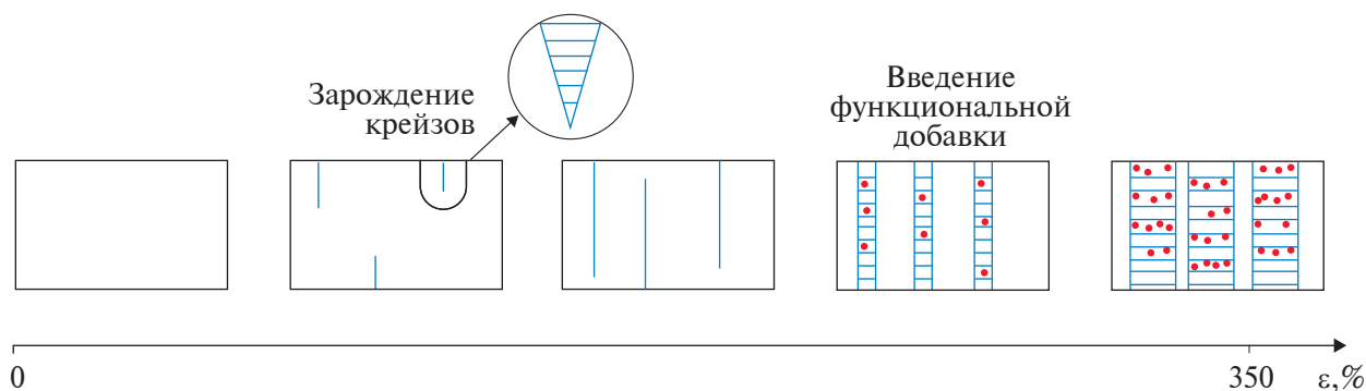
Рис. 1. Схематическое изображение структурной модификации ПЛ с одновременной импрегнацией добавки.
