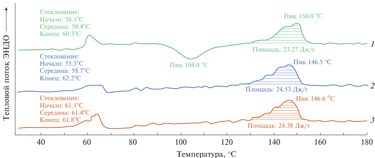
Рис. 5. ДСК-кривые первого нагрева образцов: исходный ПЛ (кривая 1), модифицированный ПЛ (кривая 2), модифицированный ПЛ с \text{CuSO}_4 (кривая 3).
