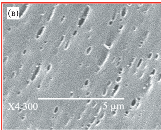
Рис. 3. СЭМ-микрофотографии ПЛ после структурной модификации с импрегнацией \text{CuSO}_4 . Микрофотография (в) является увеличенным изображением прямоугольной области, обозначенной на микрофотографии (б). Стрелками указано направление растяжения.
