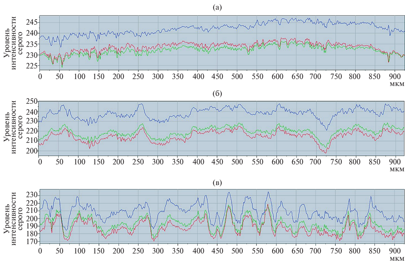
Рис. 7. Линейный профиль, полученный с помощью оптического микроскопа, образцов исходного ПЛ (а), модифицированного ПЛ без (б) и с импрегнацией CuSO_4 (в).
