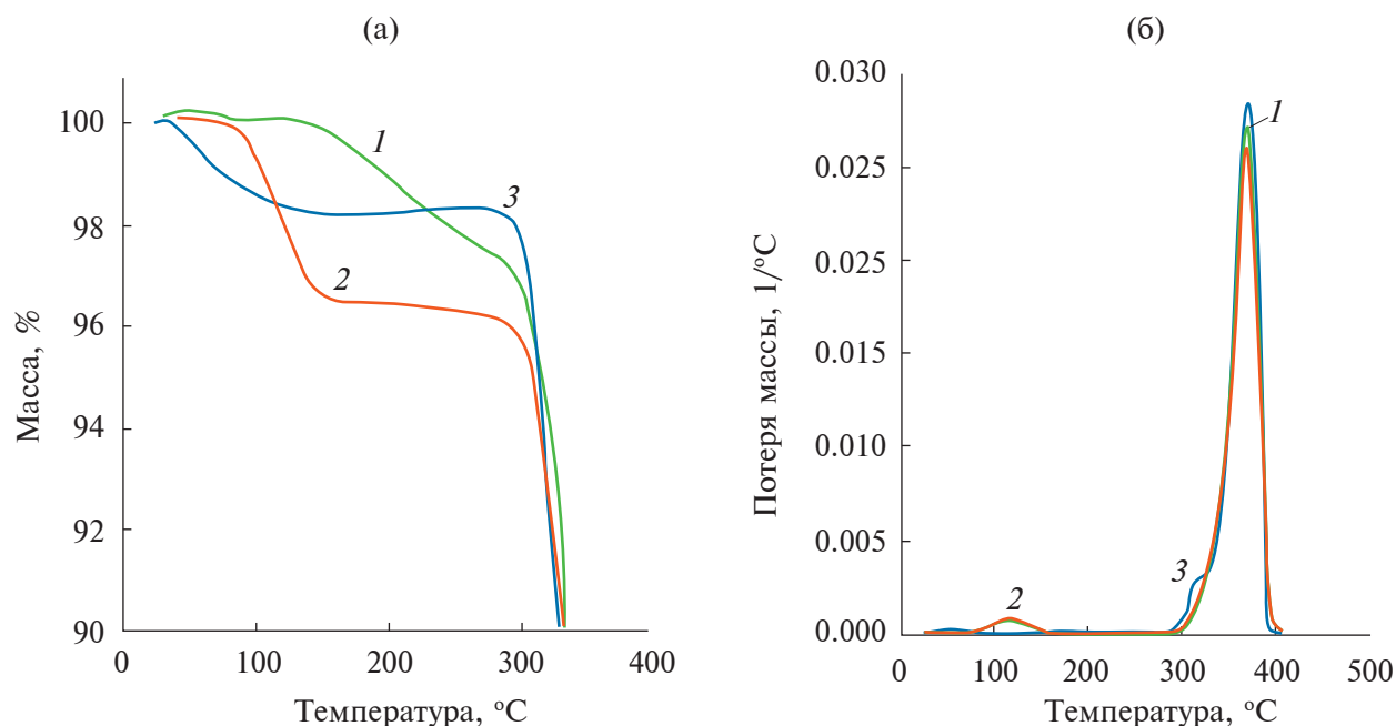
Рис. 4. Термогравиметрические (а) и дифференциальные термогравиметрические (б) кривые образцов: исходного PLL (кривая 1), модифицированного PLL (кривая 2), модифицированного PLL с \text{CuSO}_4 (кривая 3).
