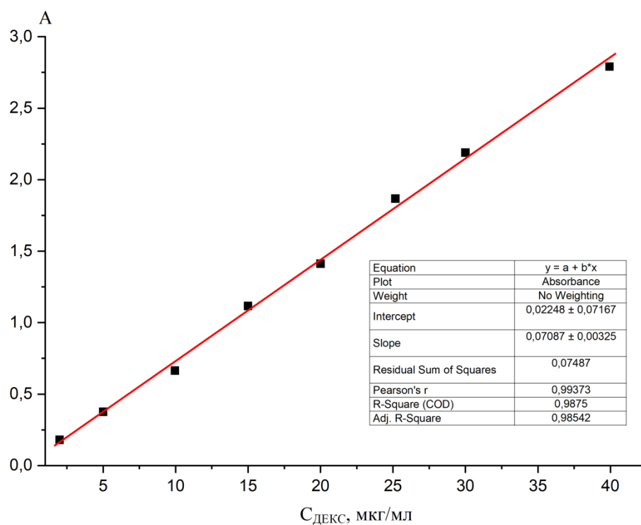
Рис. П1. Калибровочная зависимость оптической плотности раствора ДЕКС в присутствии БСА (25 мкг/мл) от концентрации ДЕКС при \lambda = 250 нм
